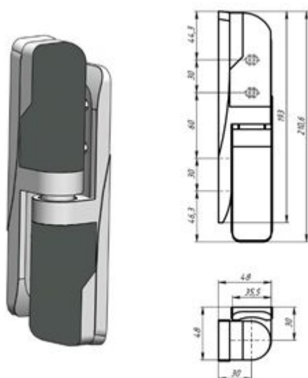
Общий вид петли в сборе
