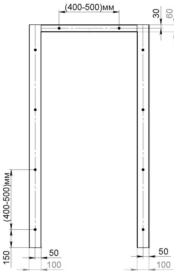
Рисунок 11. Разметка крепежных отверстий на раме
