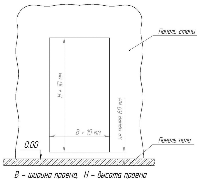
Рисунок 6. Световой проем для двери с порогом
