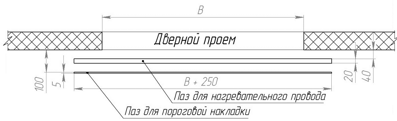
Рисунок 10. Пазы для нагревательного провода и пороговой накладки
